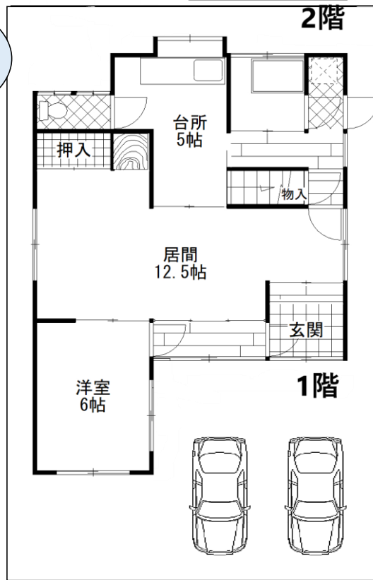
間取り図
